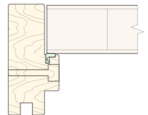
Profil av kompakt dør
