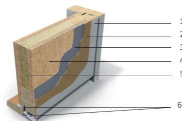
BRANNDØR (62mm) TREND TETT SLETT EI30/35DB
