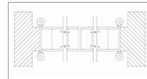
Profil av tofløyet pendelør
