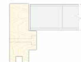
Profil av kompakt dør
