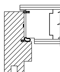
Profilbilde av B30/40dB dør. Dørbladtykkelse 58 mm.
