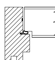
Profilbilde av B30/35dB dør. Dørbladtykkelse 52 mm.
